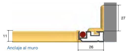
Anclaje al muro Wall fixing clip
