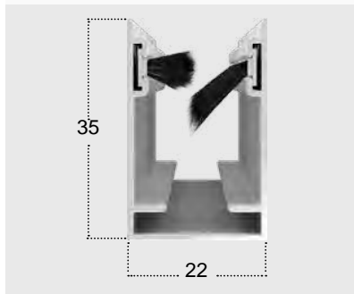
FELPUDO ANTI VIENTO ANTI WIND GUIDE
