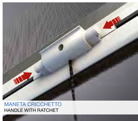
FRENO RECOGIDA LENTA "ADAGIO" Anchura mín. 650 mm "ADAGIO" BRAKE FOR SPRING min. width 650 mm
